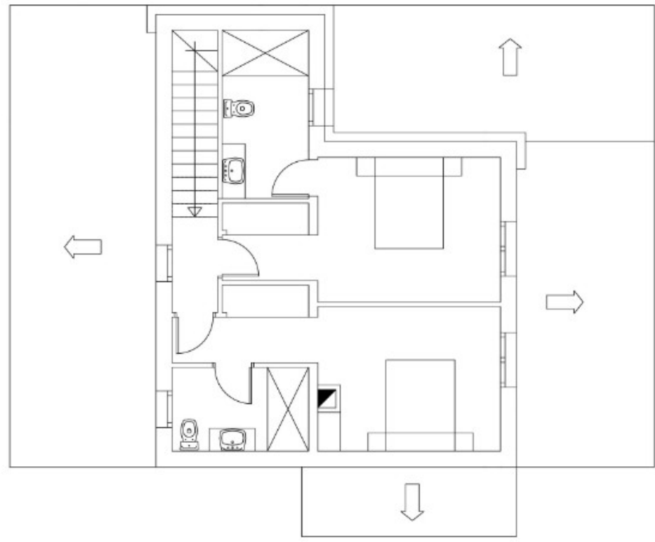
PLANTA ALTA
